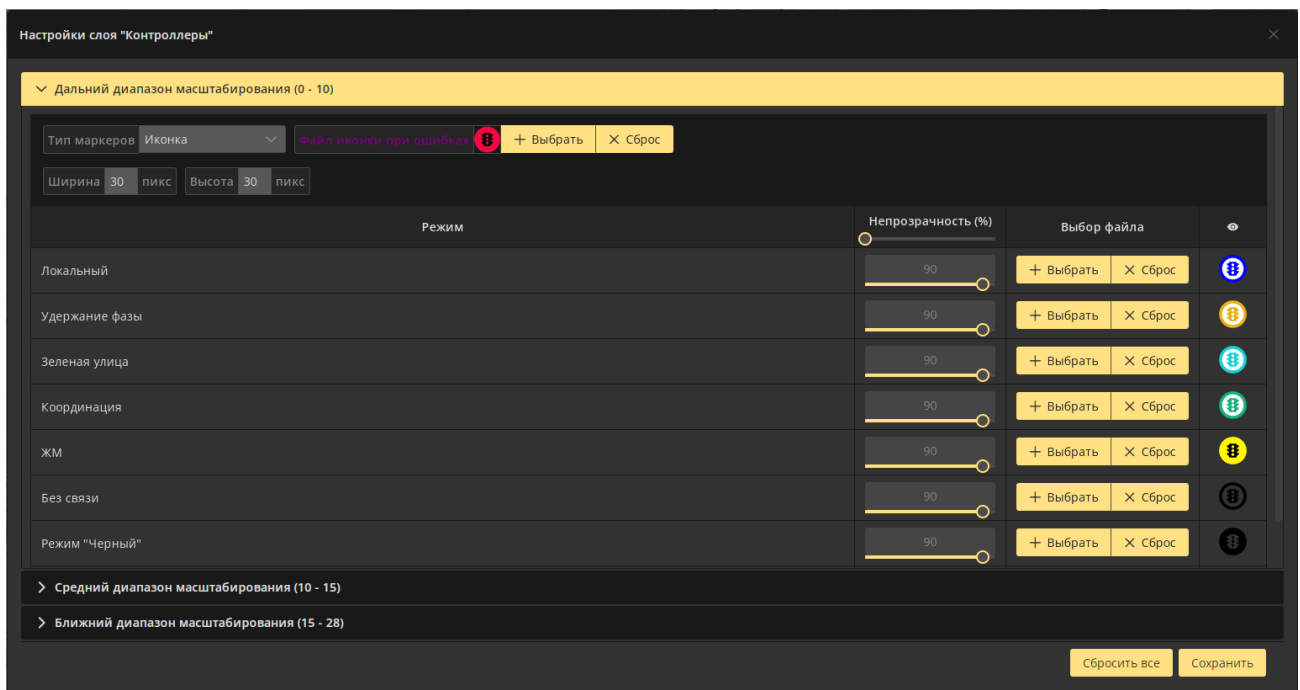
Рисунок 4.1.18 – «Настройка» слоя
