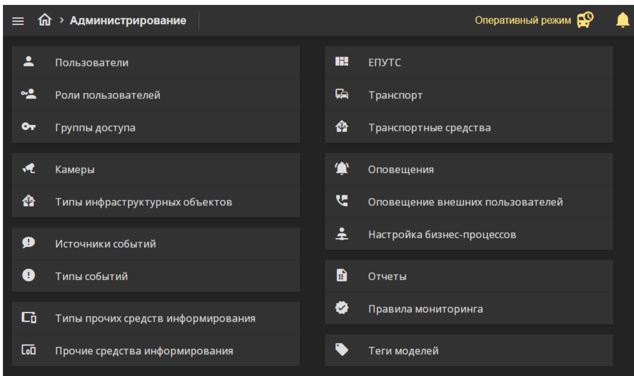
Рисунок 4.2.1– Меню «Администрирование»
